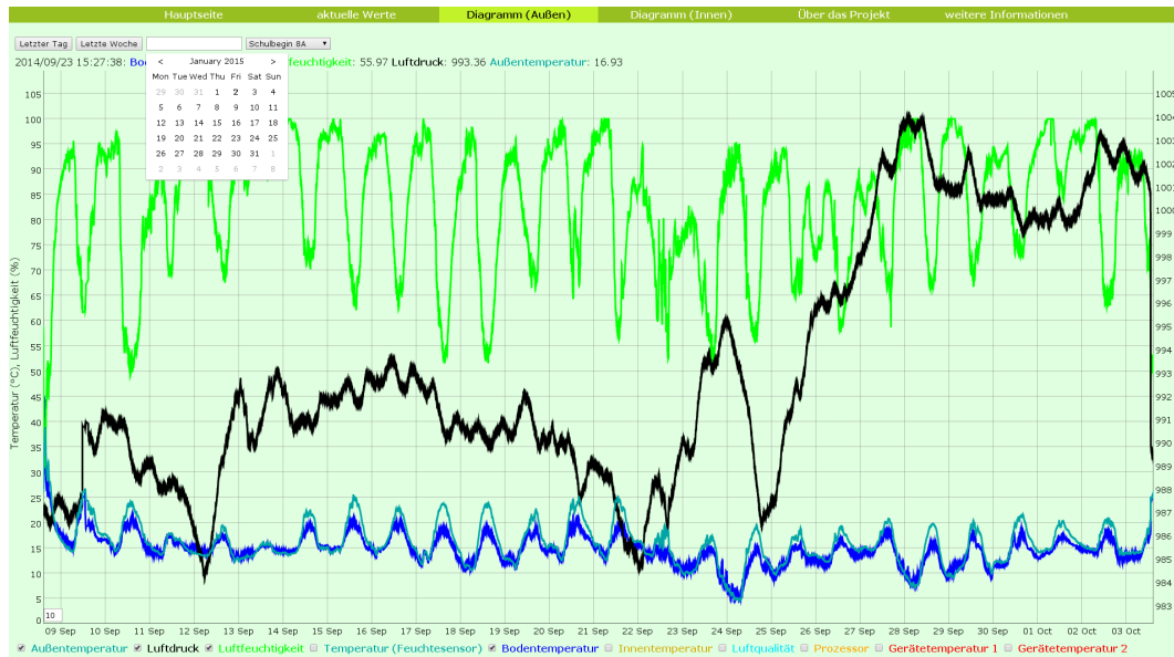
Abbildung 3.6.: Webinterface (von winkler.kremszeile.at/dygraphs_aussen.html )
