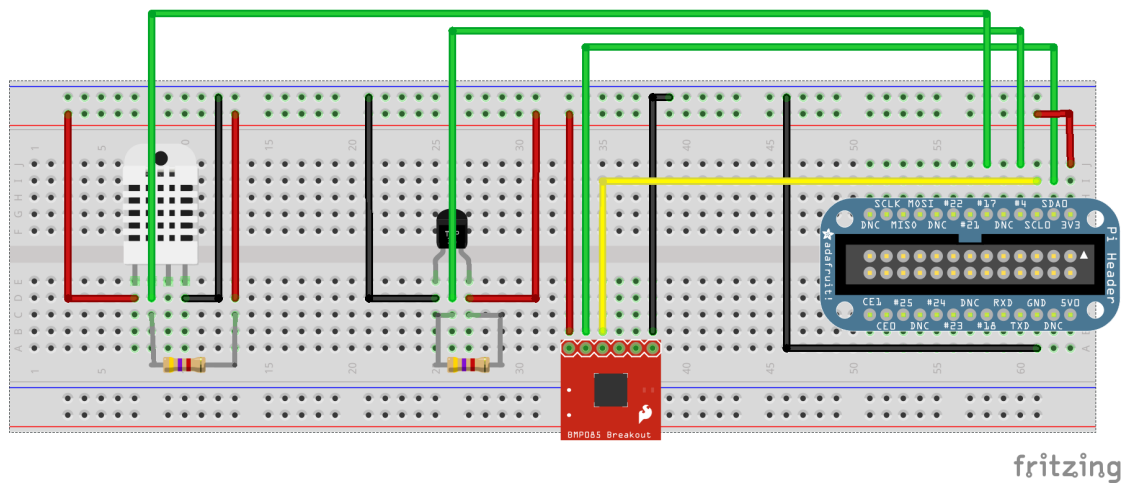
Abbildung 2.4.: Anschlusskizze von DS18B20 (Mitte; 2.2.1), DHT22 (Links; 2.2.2) und BMP085 (Rechts; 2.2.3)
