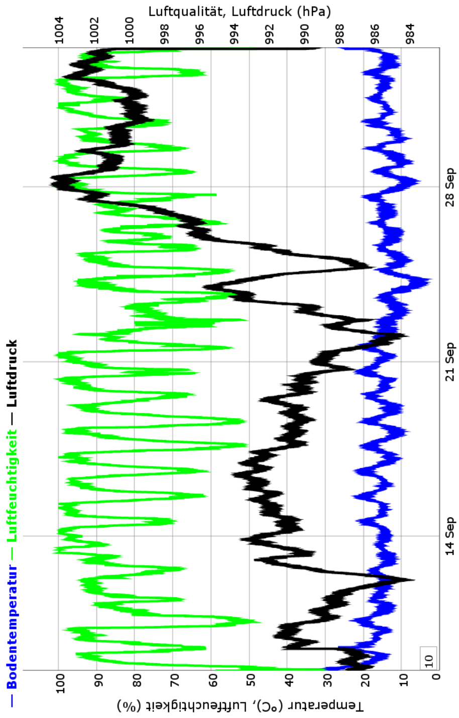
Abbildung 4.1.: Außensensoren
