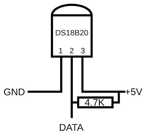
Abbildung 2.2.: Pinbelegung des DS18B20
