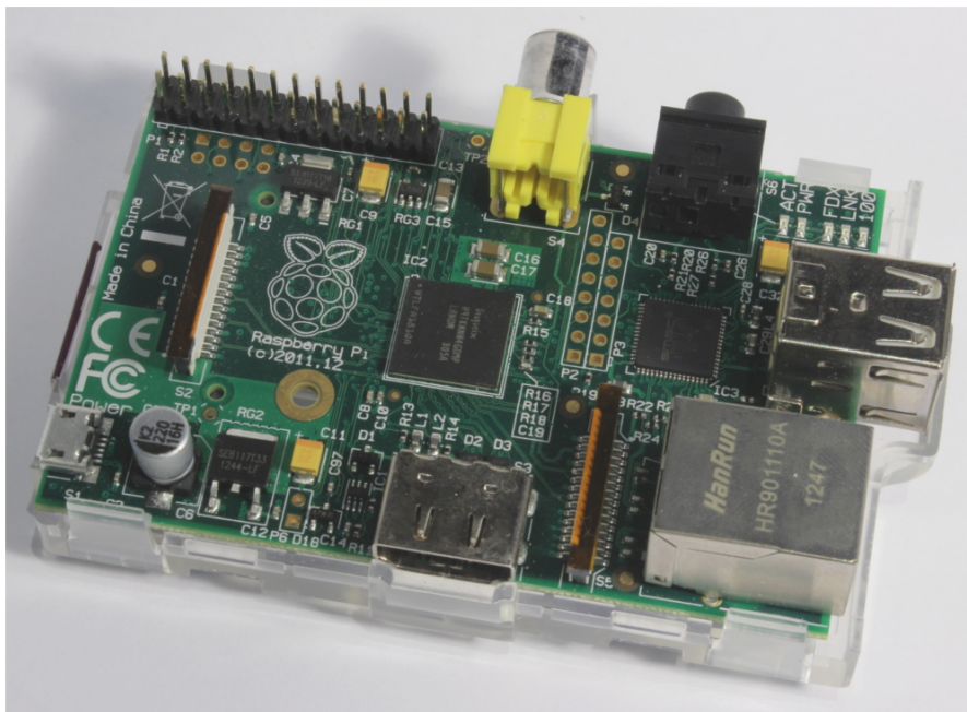
Abbildung 2.1.: Raspberry Pi - Modell B
