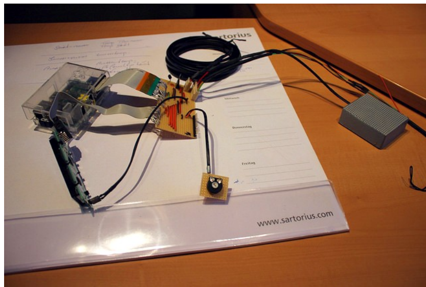
Abbildung 2.15.: Komplette Hardware
