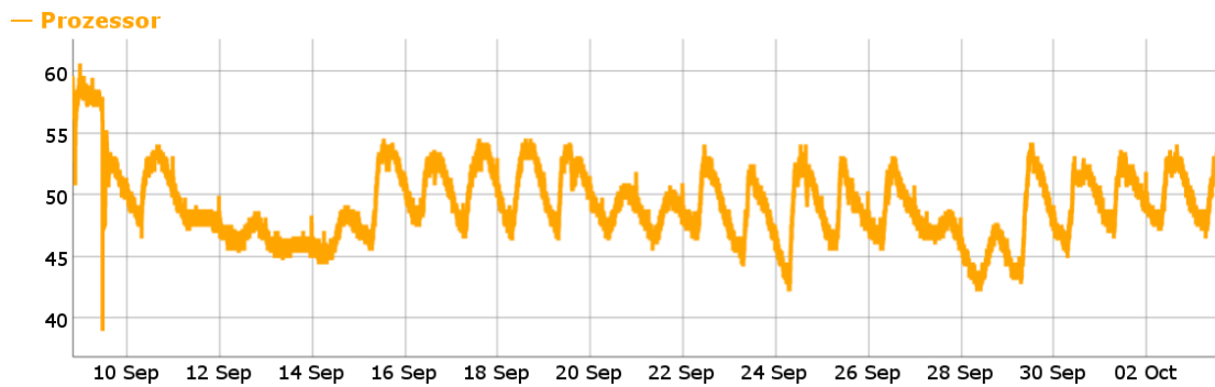
Abbildung 4.3.: CPU-Temperatur
