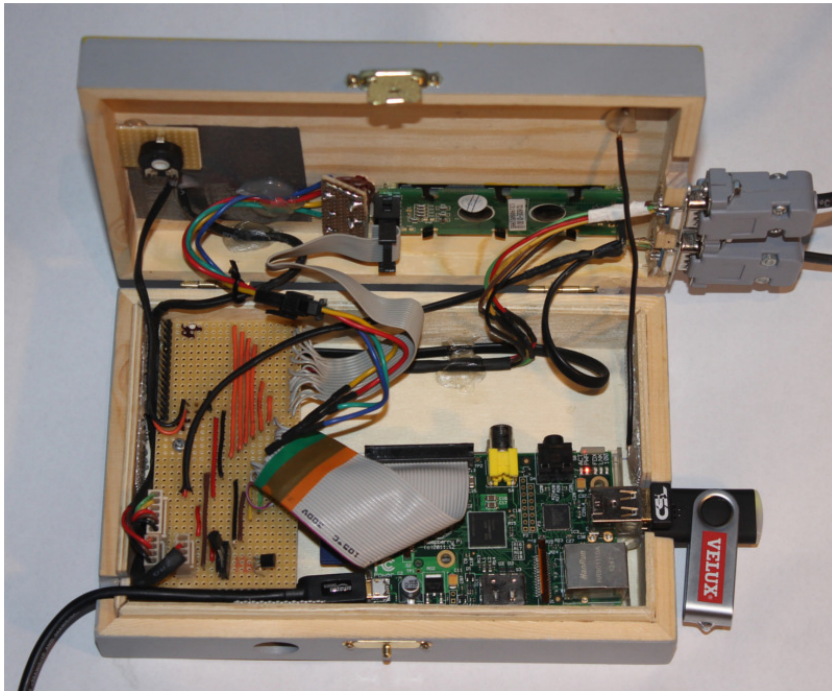
Abbildung 2.16.: Die Hardware in der Holzbox
