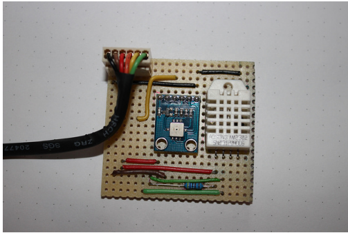
Abbildung 2.11.: Außensensoren
