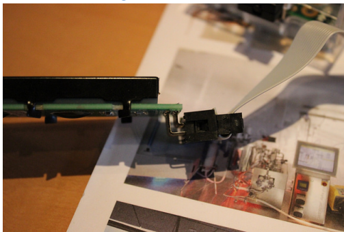
Abbildung 2.13.: Steckverbindung am Display
